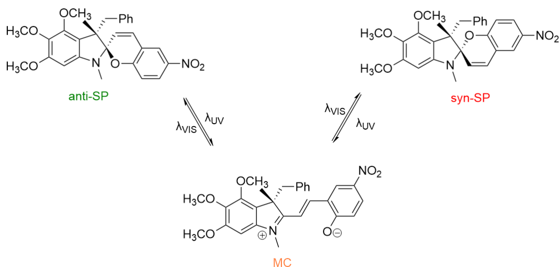
Obrázek: Rovnováha epimerního páru spiropyranu.
